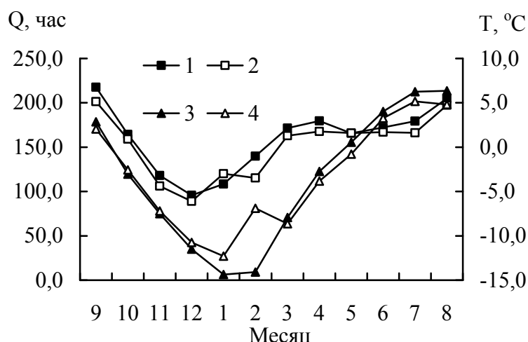
Рис. 3. Ход метеозлементов на леднике Туйыксу. 1 – продолжительности солнечного сияния (Q, час) в неблагоприятные годы; 2 – продолжительности солнечного сияния в благоприятные годы; 3 – среднемесячная температура воздуха (T, °C) в неблагоприятные годы; 4 – среднемесячная температура воздуха в благоприятные годы.
