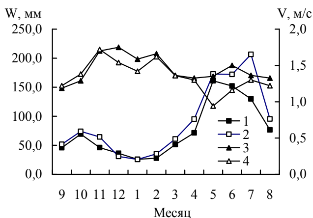
Рис. 2. Ход метеозлементов на леднике Туйыксу. 1 – суммы осадков ( W , мм) в неблагоприятные годы; 2 – суммы осадков в благоприятные годы; 3 – скорость ветра ( V , м/с) в неблагоприятные годы; 4 – скорость ветра в благоприятные годы.
