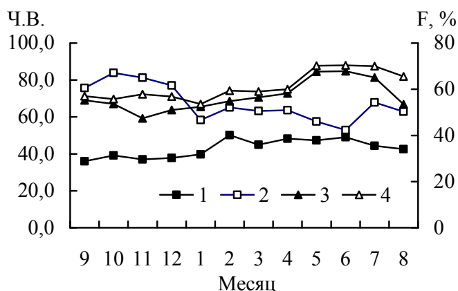
Рис. 1. Ход метеозаэлементов на леднике Туйыксу. 1 – солнечная активность (числа Вольфа) в неблагоприятные годы; 2 – солнечная активность в благоприятные годы; 3 – относительная влажность (F, %) в неблагоприятные годы; 4 – относительная влажность в благоприятные годы.
